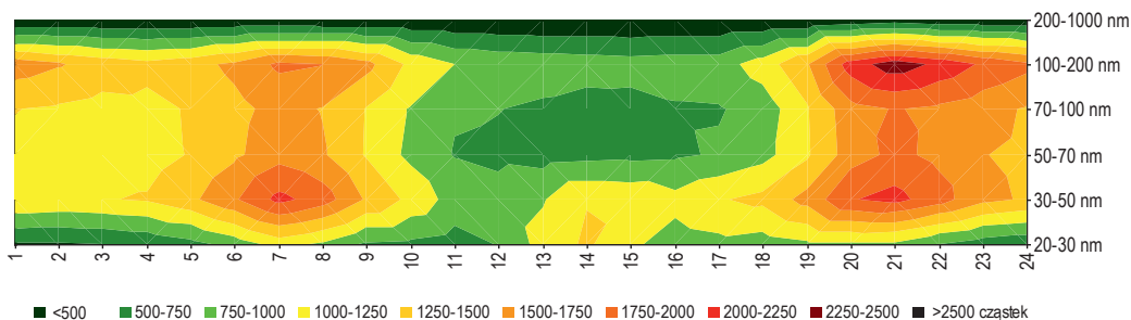
Rysunek 5-6. Rozkład średnich jednogodzinowych liczebności cząstek (liczba cząstek z sześciu różnych przedziałów wielkości: 20-30 nm, 30-50 nm, 50-70 nm, 70-100 nm, 100-200 nm i 200-1000 nm w 1 m³) w ciągu doby w obszarze miejskim (wyniki uśrednione dla sezonu letniego). Ilustrację zaczerpnięto ze sprawozdania z realizacji pracy statutowej w IPIŚ PAN w roku 2010 (IPIŚ PAN, 2011).
