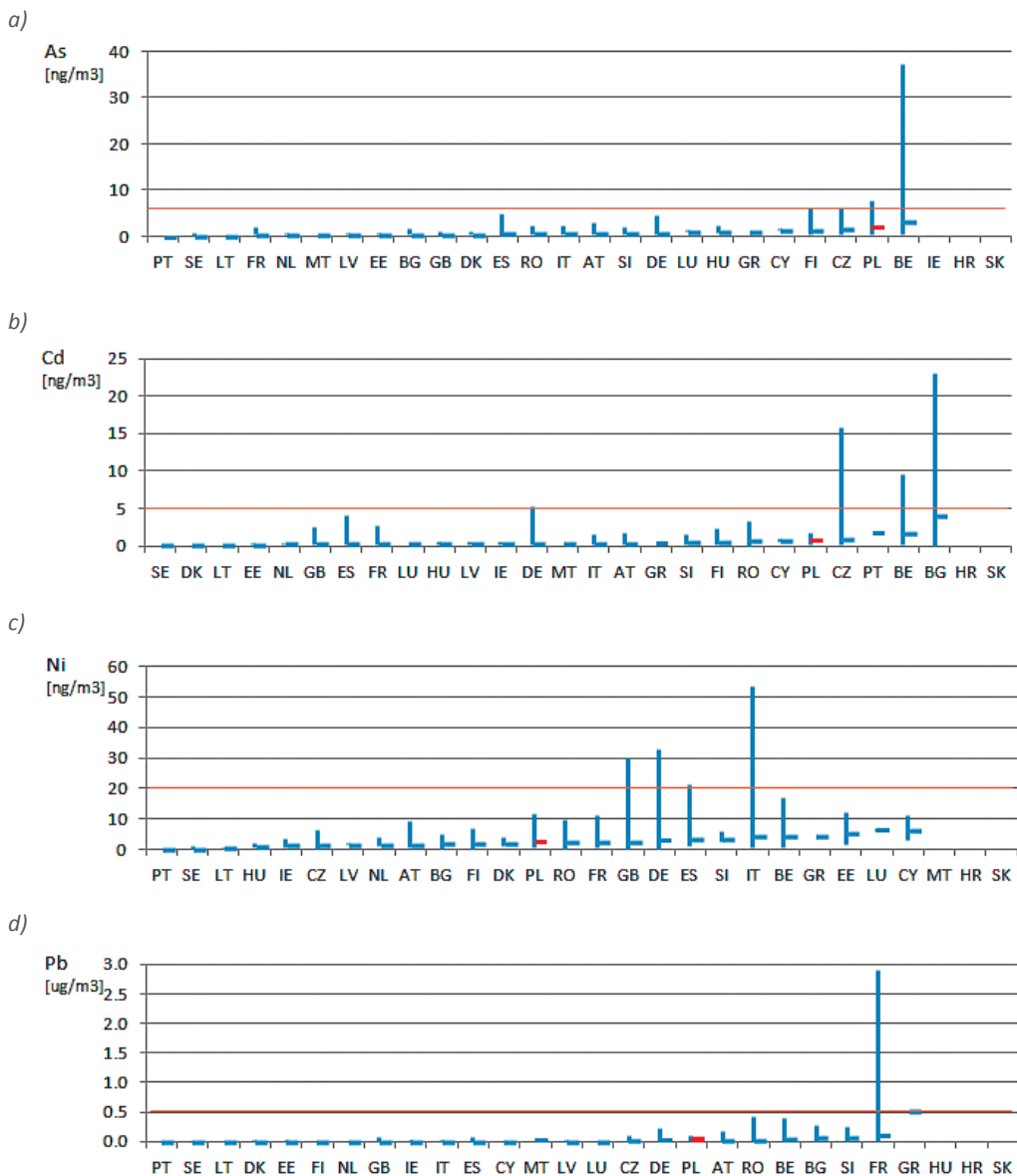
Rysunek 11.5-8. Minimalne, średnie i maksymalne stężenia a) arsenu [ \text{ng}/\text{m}^3 ], b) kadmu [ \text{ng}/\text{m}^3 ], c) niklu [ \text{ng}/\text{m}^3 ] i d) ołowiu [ \mu\text{g}/\text{m}^3 ] w krajach Unii Europejskiej w 2012 r. Źródło danych: AirBase.
