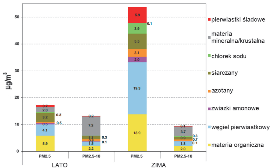
Rysunek 5-10. Składowe składniki PM 2,5 i PM 2,5-10 w obszarze miejskim. Ilustracja zaczerpnięta z pracy Roguli-Kozłowskiej i in. (2012).
