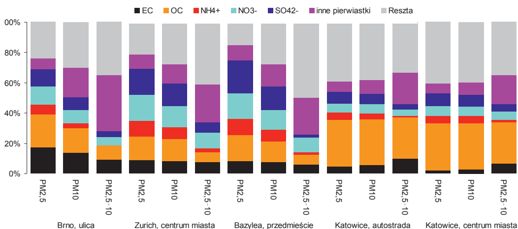
Rysunek 5-12. Udział procentowy składników chemicznych i grup składników chemicznych (pierwiastki) w masie PM w różnych lokalizacjach, dla trzech frakcji PM. Opracowanie własne danych zaczerpniętych z publikacji Hüeglina i in. (2005) i Roguli-Kozłowskiej (2014).
