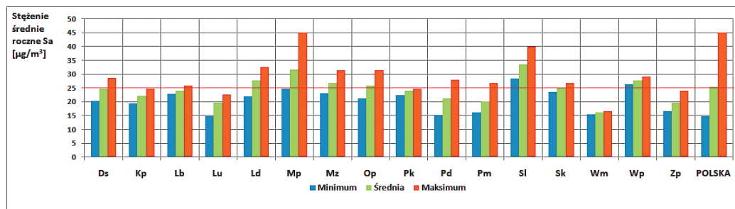
Rysunek 11.1-5. Wartości minimalna, średnia i maksymalna stężenia średniego rocznego PM 2,5 w 2014 r. dla każdego województwa i dla kraju, obliczone na podstawie serii pomiarów stężeń pyłu PM 2,5 ze stanowisk tła miejskiego i podmiejskiego (skrótów nazw województw podane są w tabeli 11.1-3). Źródło: opracowanie własne na podstawie danych PMŚ.
