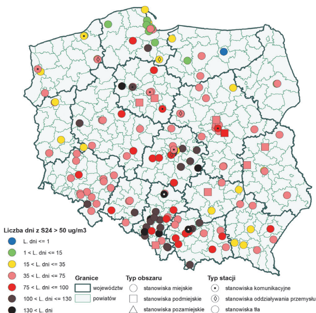
Rysunek 11.1-4. Liczba dni w 2014 r. ze stężeniem 24-godz. pyłu PM10 wyższym od 50 \mu\text{g}/\text{m}^3 na podstawie pomiarów na stanowiskach miejskich i podmiejskich. Źródło: opracowanie własne na podstawie danych PMŚ.
