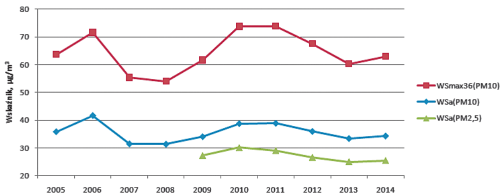
Rysunek 11.1-9. Wartości wskaźników WSmaks36(PM10), WSa(PM10) i WSa(PM2,5) w kolejnych latach. Opracowanie własne na podstawie danych PMŚ.
