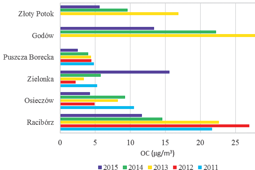
Rysunek 11.4-26. Stężenie OC [ \mu\text{g}/\text{m}^3 ] w sezonie a) niegrzewczym, b) grzewczym. Opracowanie własne, źródło danych PMŚ, IPIŚ PAN.
