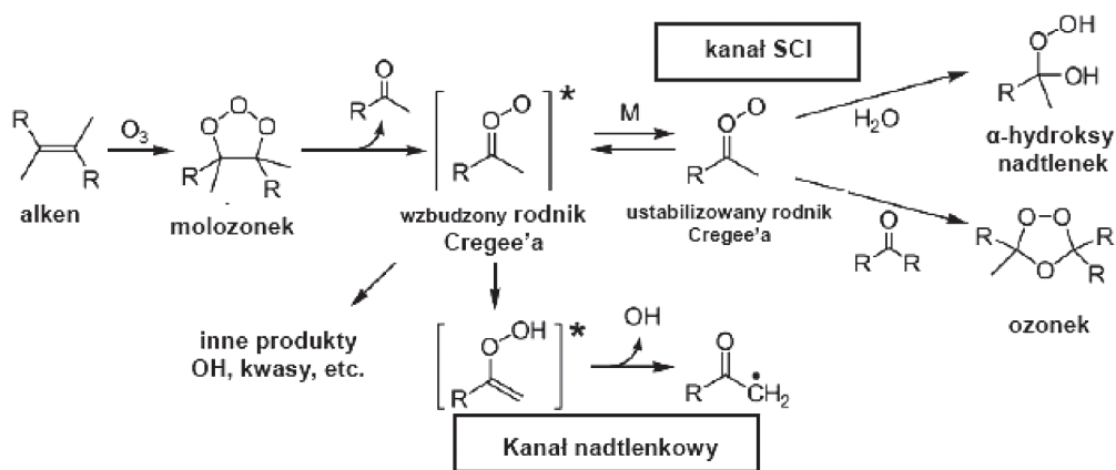
Rysunek 3.5-3. Uproszczony mechanizm reakcji alkenu z ozonem. Różne konfiguracje przestrzenne związku Criegee'a (syn oraz anti) zostały ujednoczone. Produkty o małej lotności mogą powstawać na dwa sposoby bądź w tzw. kanale nadtlenkowym lub tzw. kanale SCI. Tylko dwie możliwe reakcje w kanale SCI zostały przedstawione na rysunku. W niektórych przypadkach powstały α-hydroksy nadtlenek jest nietrwały. (SCI – stabilizowany Criegee intermediate – spowolnione rodniki Criegee'a). Źródło: Atkinson i Arey, 2003.
